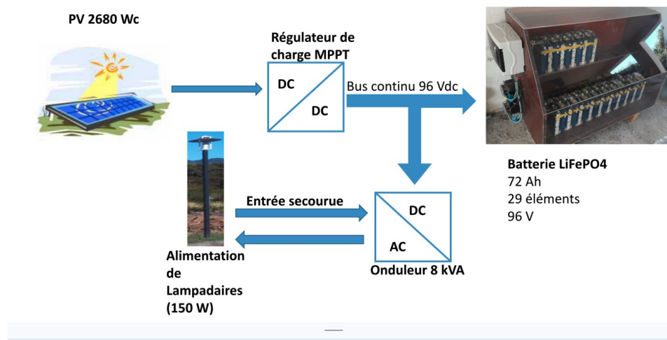
Fig.1 : Synoptique système
